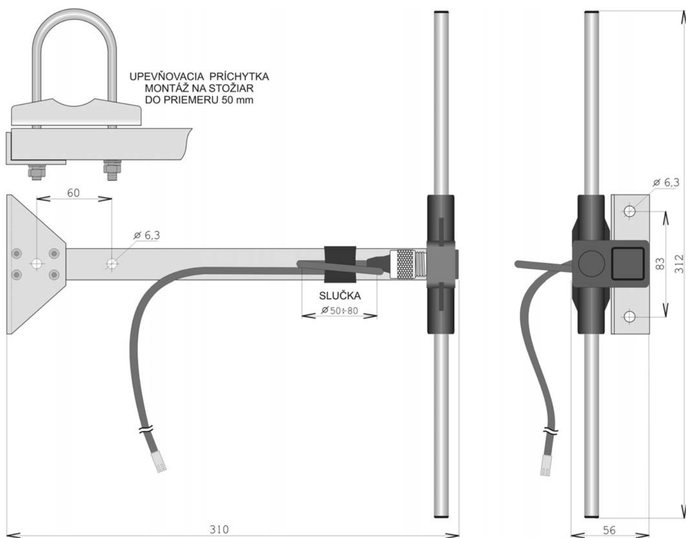
Mechanické rozmery antény AN-03
