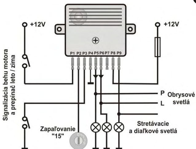
1. paralelné zapojenie
