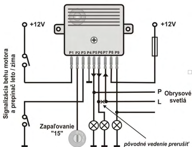
2. sériové zapojenie
