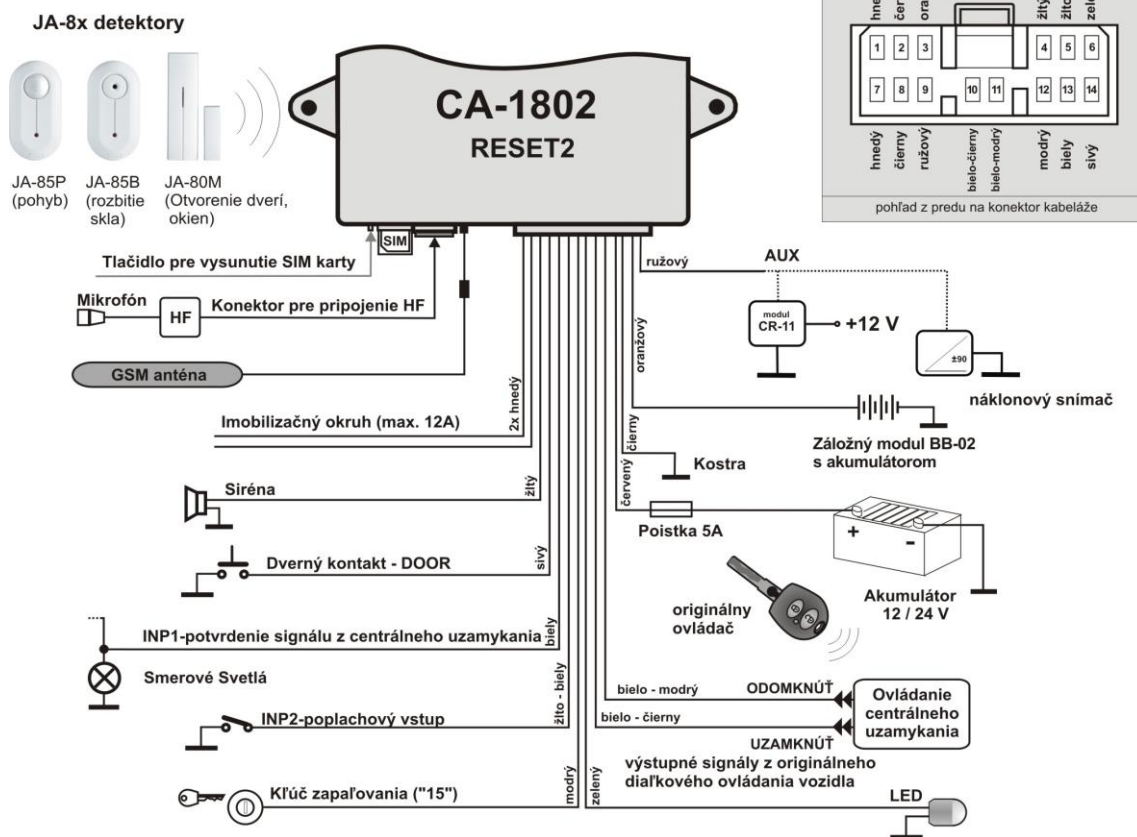
Obr. 1: Zapojenie alarmu v režime RESET 2. V tomto režime prevádzky je autoalarm ovládaný jednotkou centrálného uzamykania vozidla.
