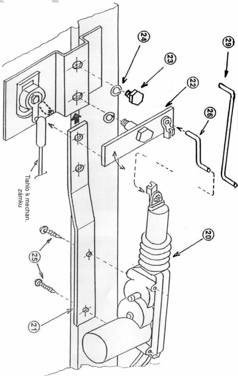
Obr.: Montáž servomotora pre 5. dvere FAVORIT (pohľad zvnútra).
