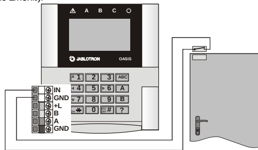
obr. 2 Príklad zapojenia detektora otvorenia dverí
