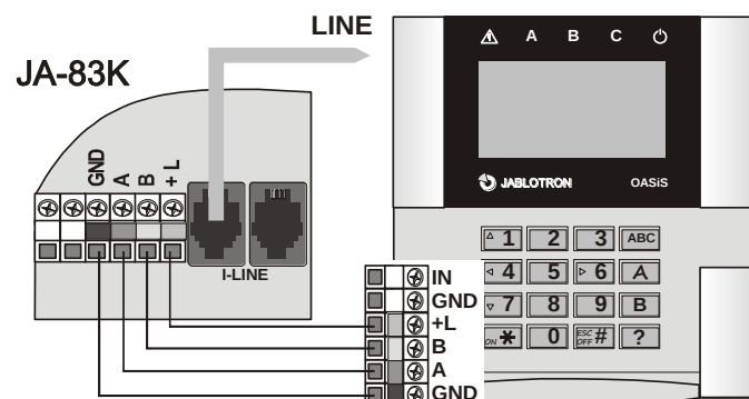
obr. 1 prepojenie klávesnice s ústredňou
