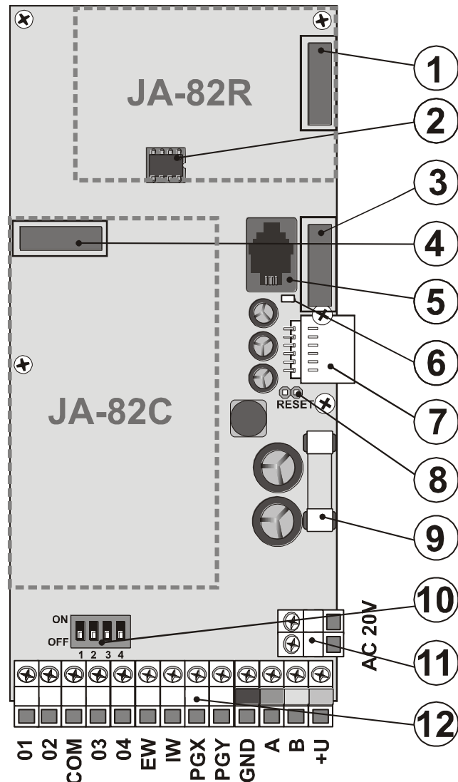
obr. 1 Elektronika ústredne
