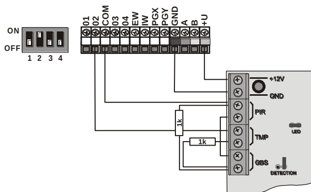
obr. 4 Zapojenie kombinovaného detektora JS-25 Combo do jednej slučky
