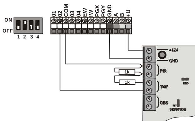
obr. 3 Zapojenie pohybového detektora JS-20 Largo
