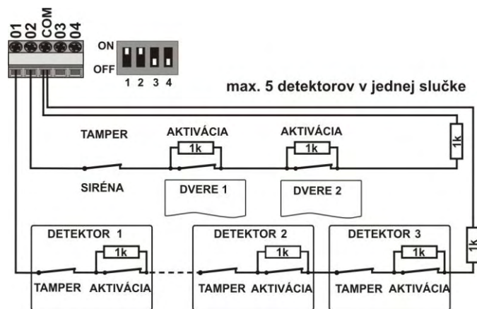
obr. 6 Zapojenie viacerých detektorov do vstupov – schematicky
