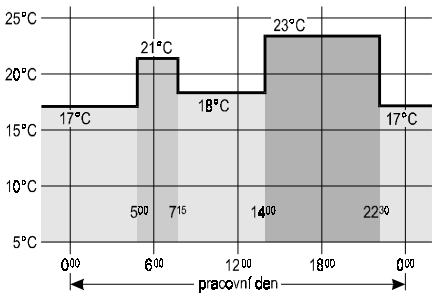
Průběh teploty dle příkladu A
